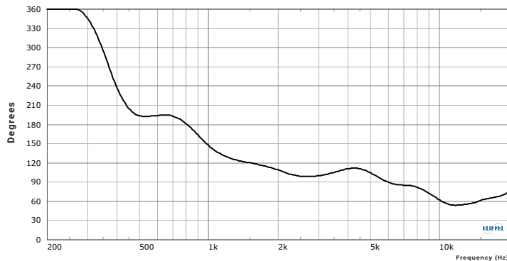
Beamwidth
