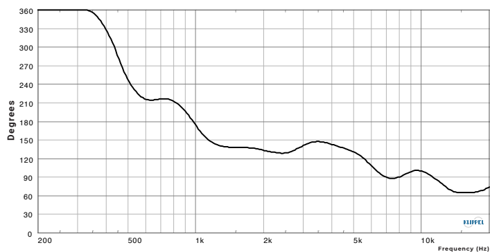
Beamwidth
